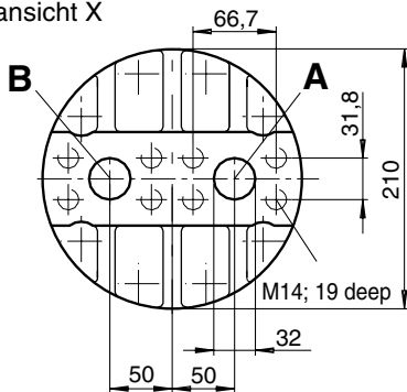
Teilansicht X
